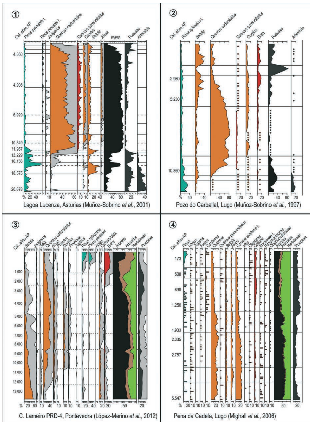
Figura 6. 1–4, Expansión de vegetación xerofítica durante el Dryas reciente, dando paso a formaciones arbóreas de pinar con abedul y finalmente sustitución hacia bosques de Quercus caducifolia durante el Holoceno. Cal., calibrados; AP, Antes del Presente; PA, Polen Arbóreo; PNA, Polen No Arbóreo. Secuencias extraídas de Carrión et al. (2015) y redibujadas de las citas indicadas.
