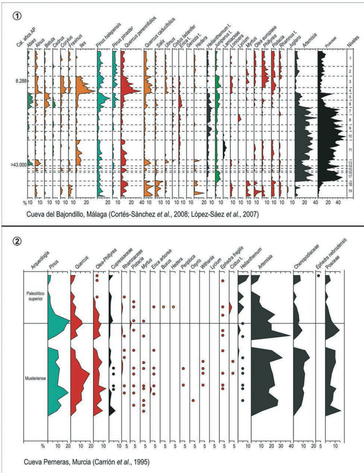
Figura 5. 1–2, Elementos leñosos templados, mediterráneos e ibero-magrebíes del litoral mediterráneo peninsular en el Pleistoceno. Secuencias extraídas de Carrión et al. (2015) y redibujadas de las citas indicadas.
