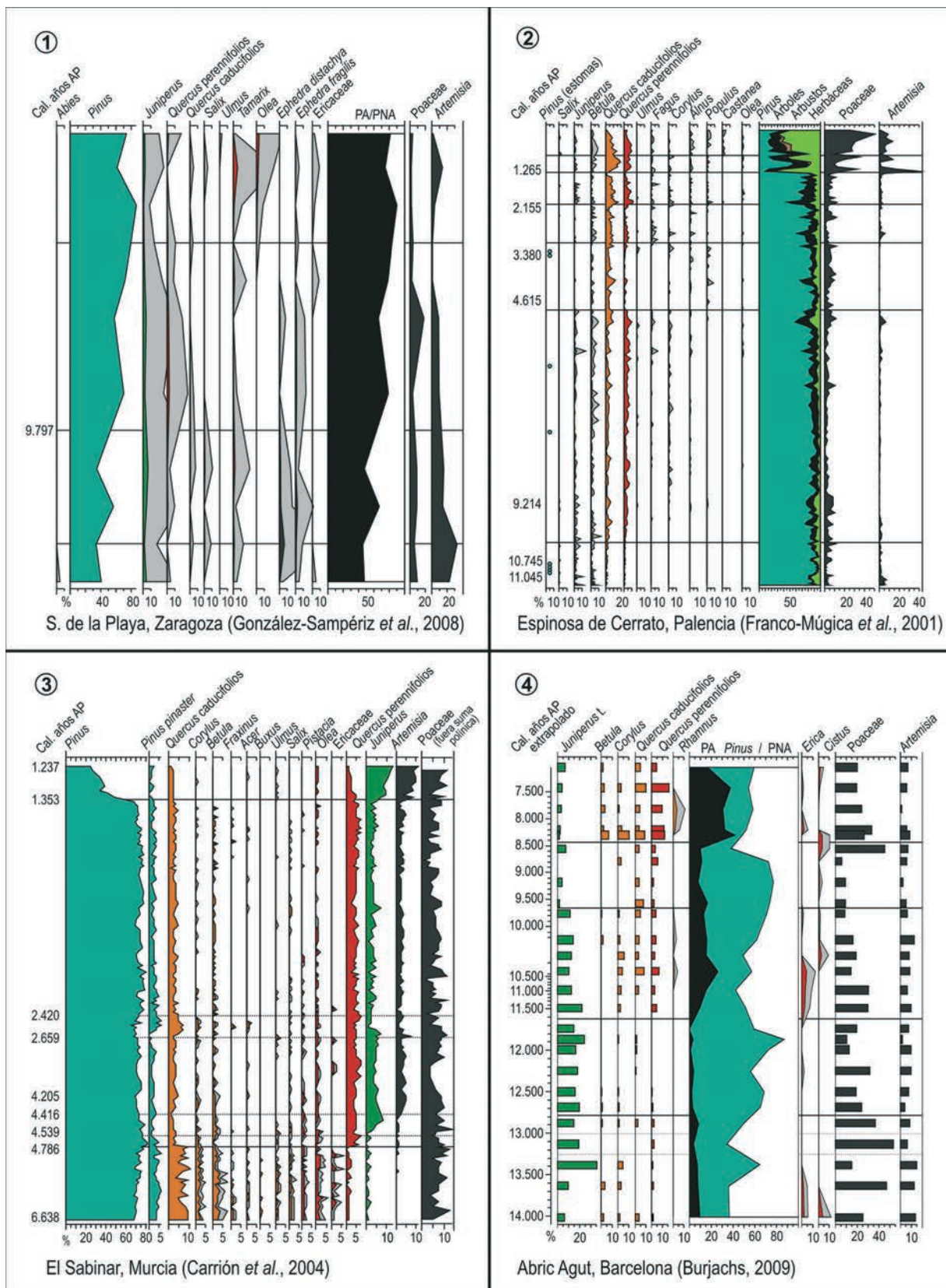
Figura 7. 1–4, Registros ibéricos en los que domina el bosque de pinar durante la mayor parte del Holoceno. Cal. , calibrados; AP , Antes del Presente; PA , Polen Arbóreo; PNA , Polen No Arbóreo. Secuencias extraídas de Carrión et al. (2015) y redibujadas de las citas indicadas.
